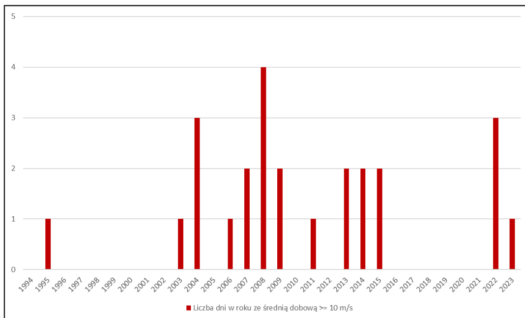
Rysunek 24. Liczba dni w roku z dobową prędkością wiatru \geq 10 m/s w Rawiczu w latach 1994–2023
