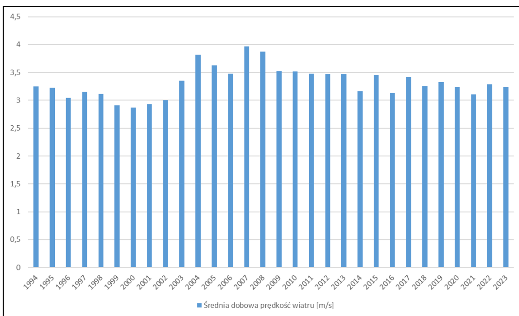
Rysunek 23. Średnia dobowa prędkość wiatru w układzie rocznym Rawiczu w latach 1994–2023
