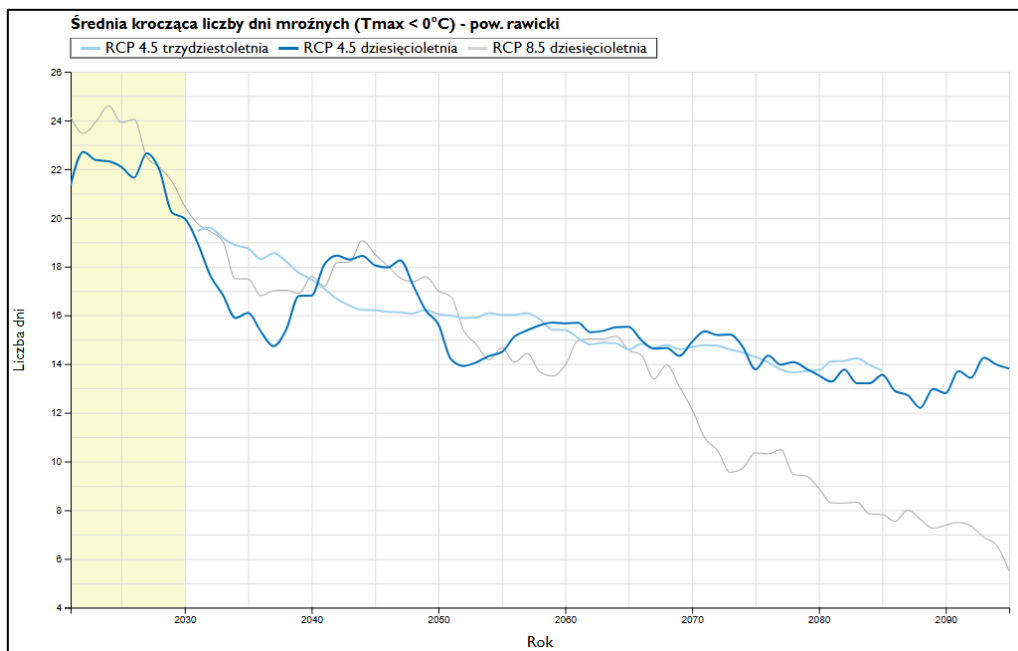
Rysunek 32. Prognoza zmian liczby dni mroźnych ( T_{MAX} < 0^{\circ}C ) do 2100 r. w rejonie Rawicza
